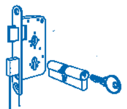
Profil-Sicherheitszylinder
